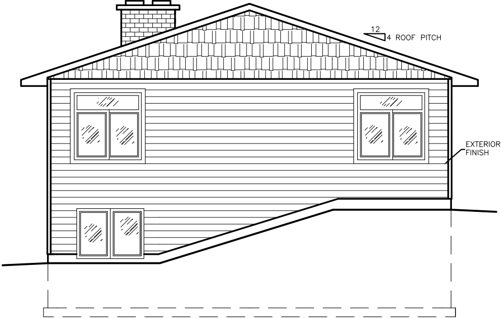
END ELEVATION
